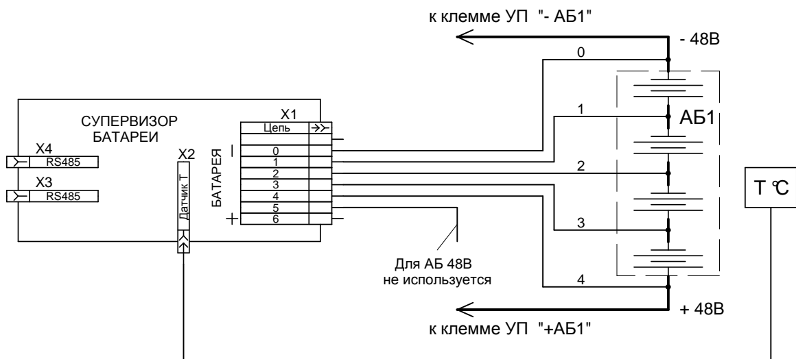
Рисунок 2.1 – Схематическое изображение подключения модуля САБ
